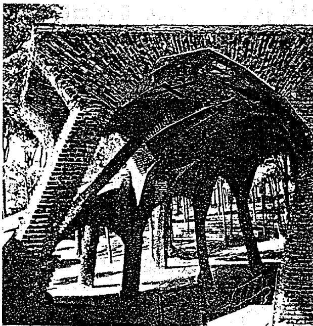
Figura 9. — El pórtico de la cripta, sostenido por pilares inclinados de ladrillo. (Foto «Amigos de Gaudí».)
