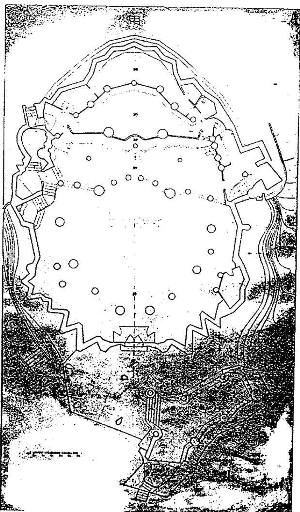
Figura 6. — Planta de la cripta de la Colonia Güell. Plano levantado por Luis Bonet Garí. (Foto «Amigos de Gaudí».)
