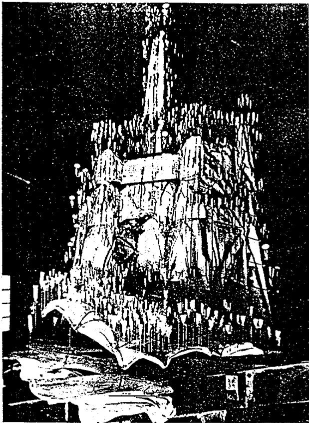
Figura 8. — Santa Coloma de Cervelló. Capilla Colonia Güell. Taller del arquitecto Gaudí. Funicula del conjunto. (Foto Mas.)
