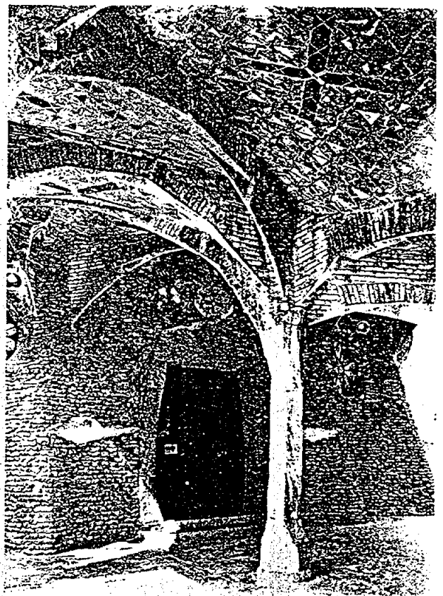
Figura 10. — El pórtico de la cripta con bóvedas tabicadas de paraboloides, hiperbólicos. (Foto «Amigos de Gaudí».)
