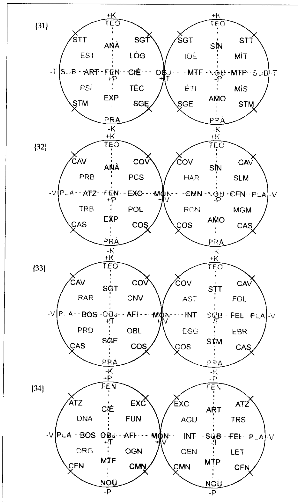
Esquema XX: Les quatre esferes canòniques de la D-3
