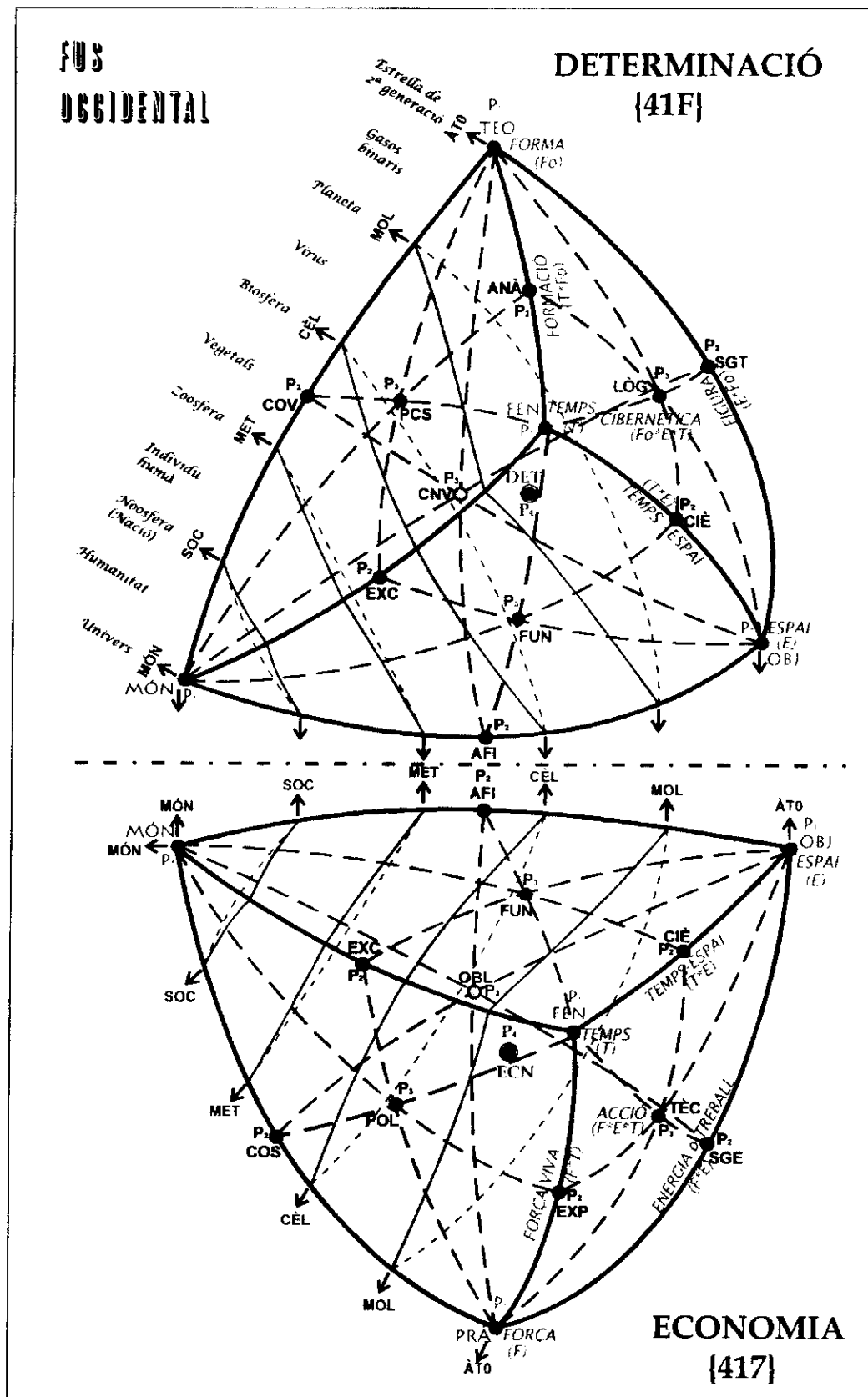
Esquema XXXIII: Exemple de dues "cambres gòtiques", tetraedres hiperesfèrics
