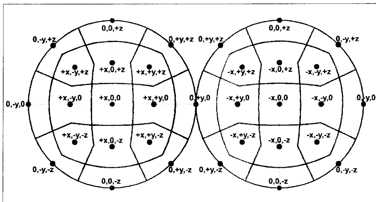
Esquema XXI: Oscil·lació superficial esfèrica
