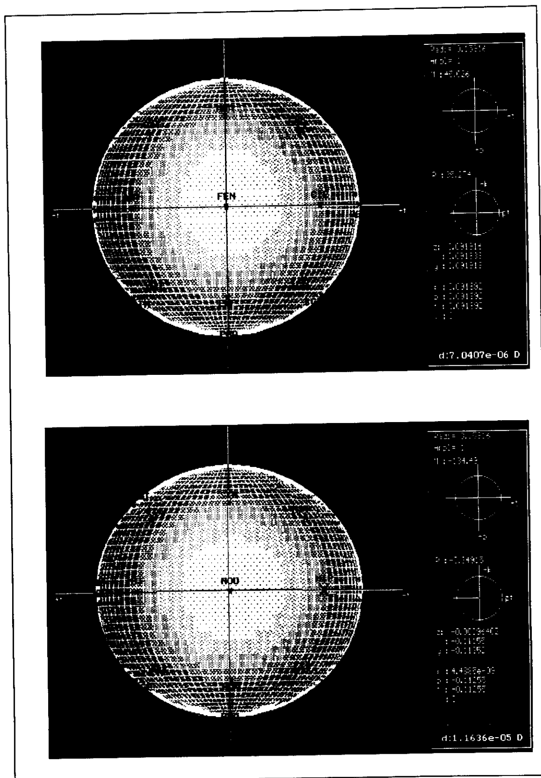
Esquema XXX: Tall esfèric de radi màxim (0,15916C) {31}. Damunt FEN (cursor en LÒG) i davall NOÛ (cursor en MTP) - segons programa "GLOBUS".
