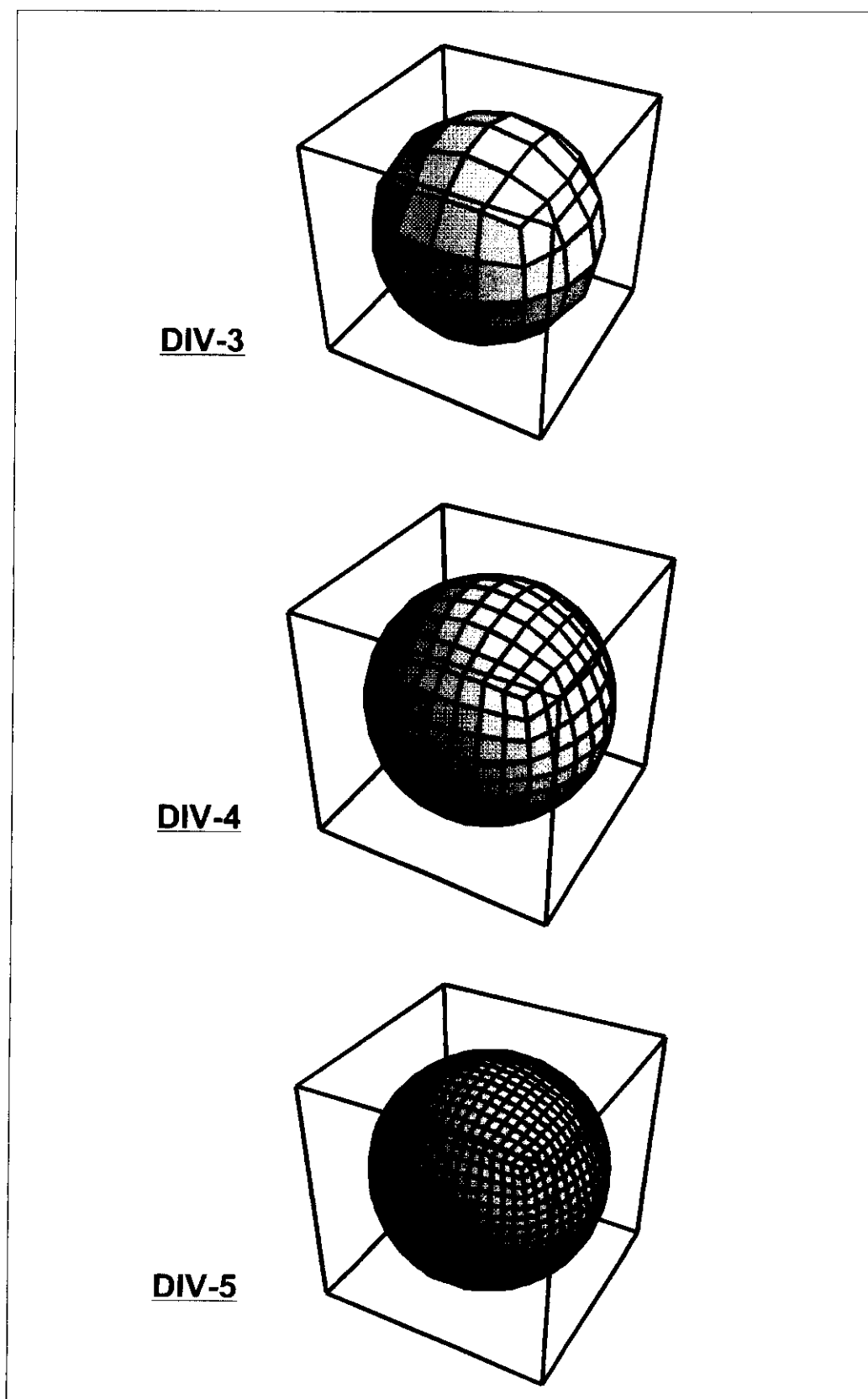
Esquema XXXIX: Divisions 3, 4 i 5 de la superfície esfèrica, segons programa de "Trigonometria Hiperesfèrica"
