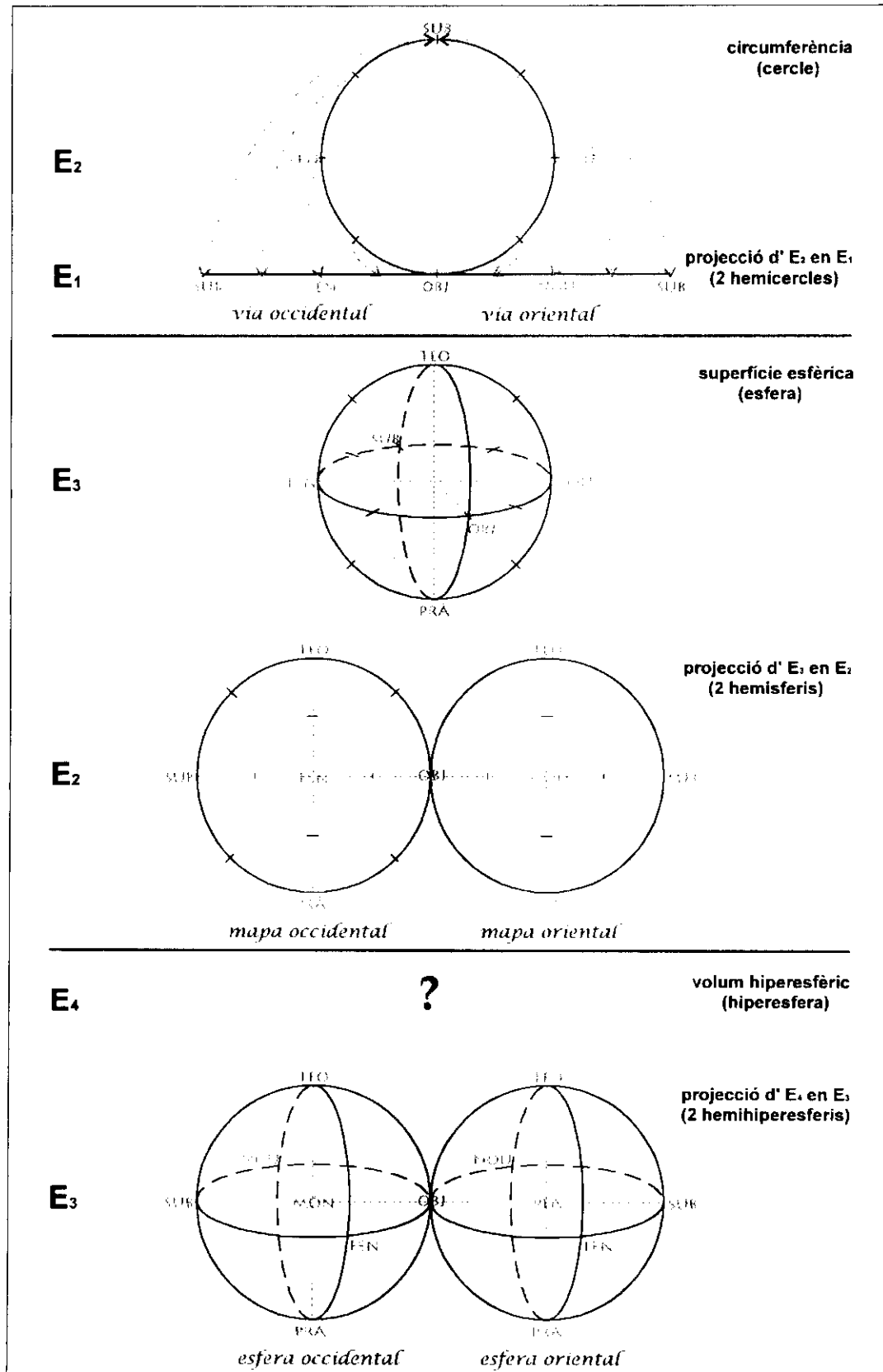
Esquema XIV: Projeccions de Globus E^N a E^{N-1}
